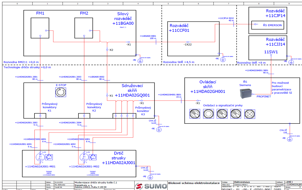
Obrázek 1 Návrh technického řešení drtičky strusky, Mělník 1
