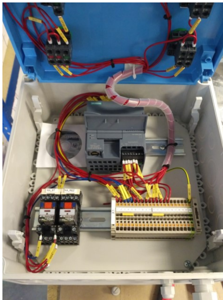
Obrázek 3 Rozvaděč 1
